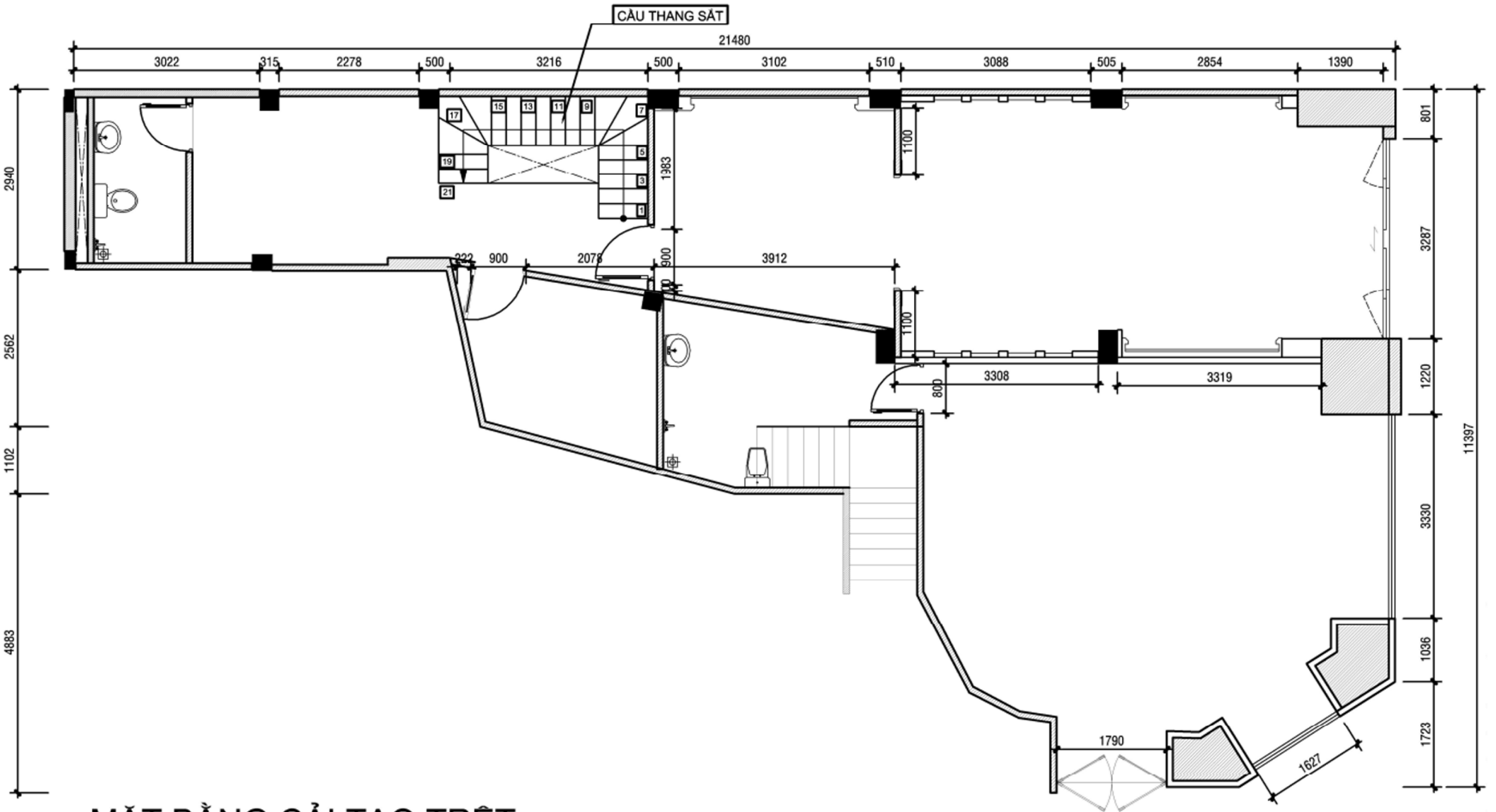
MẶT BẰNG CẢI TẠO TRỆT TL: 1/100
